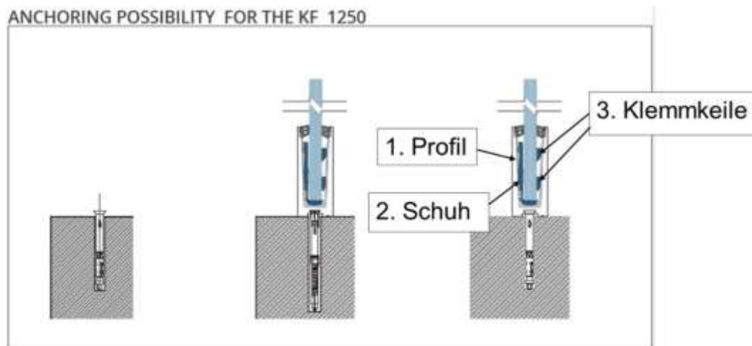
Abb. 2-6 Profil KF 1250, Übersicht
